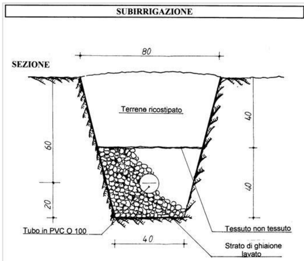
Schema subirrigazione
